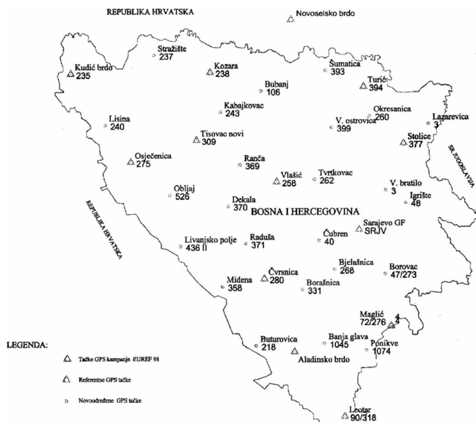
sl.1. Raspored GPS tačaka kampanje BIHREF2000
