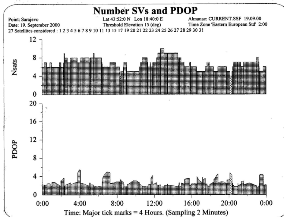
SI.2. Broj i raspored satelita i PDOP tokom kampanje BIHREF2000
